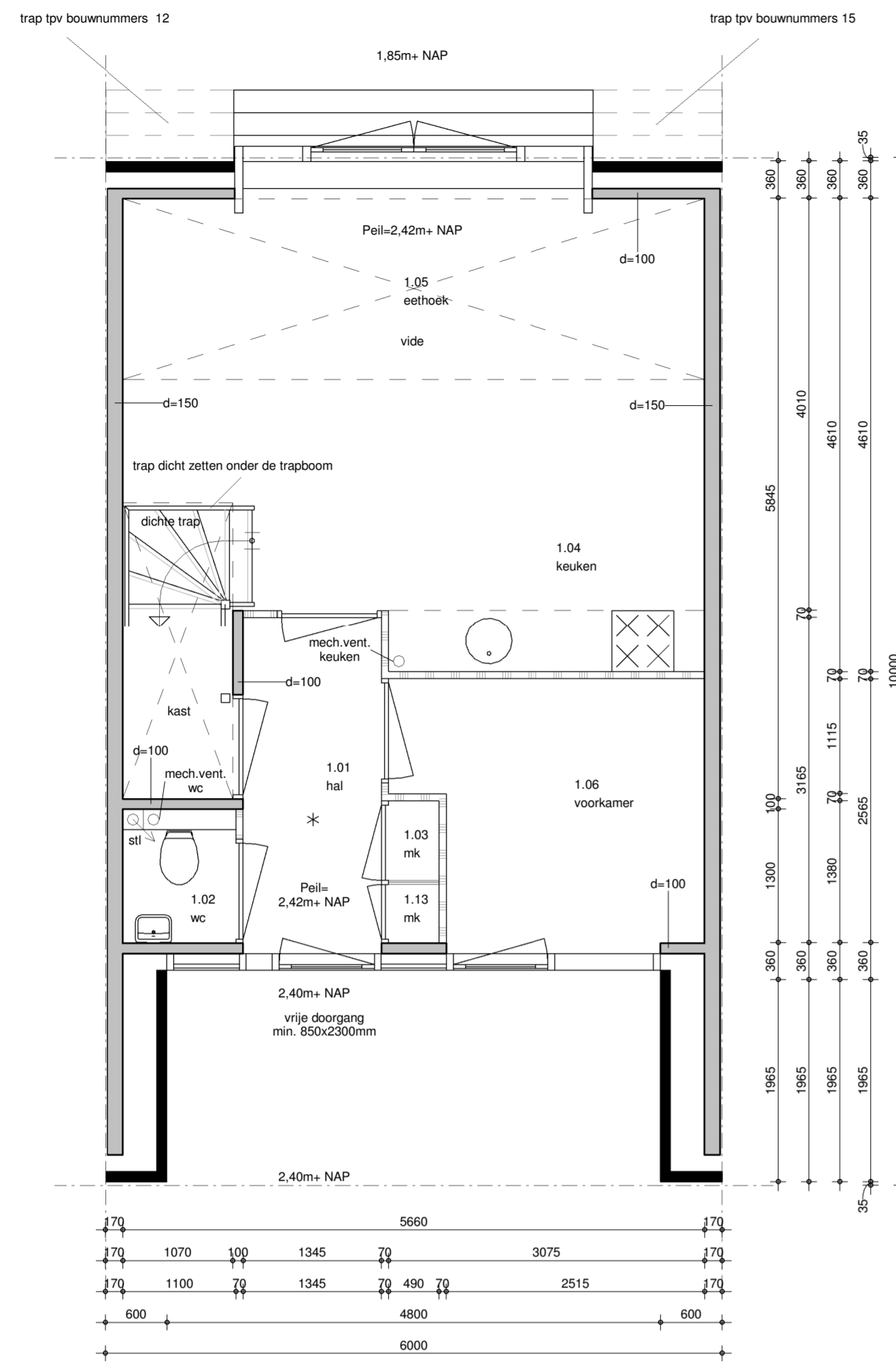
begane grond 1 : 50
