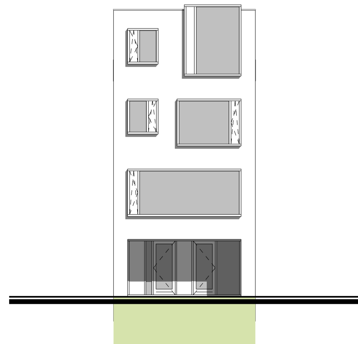
voorgevel 1 : 100
