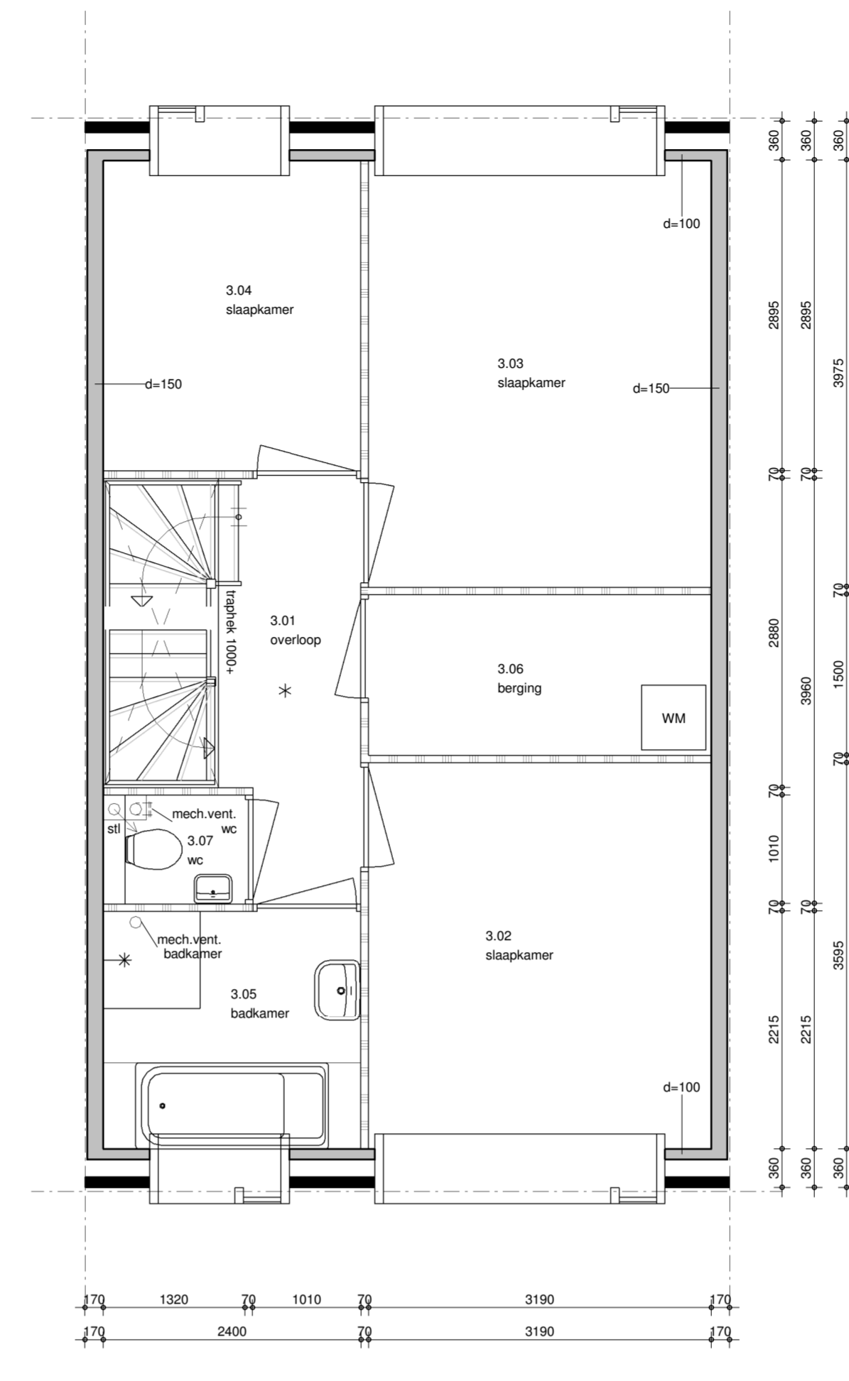
tweede verdieping 1 : 50
