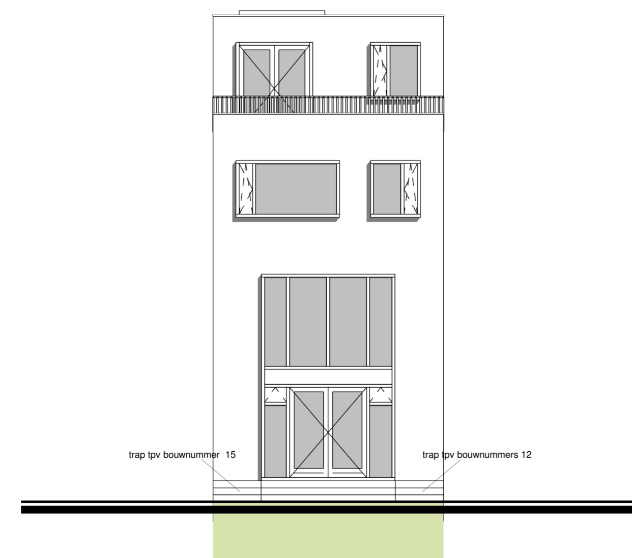
achtergevel 1 : 100
