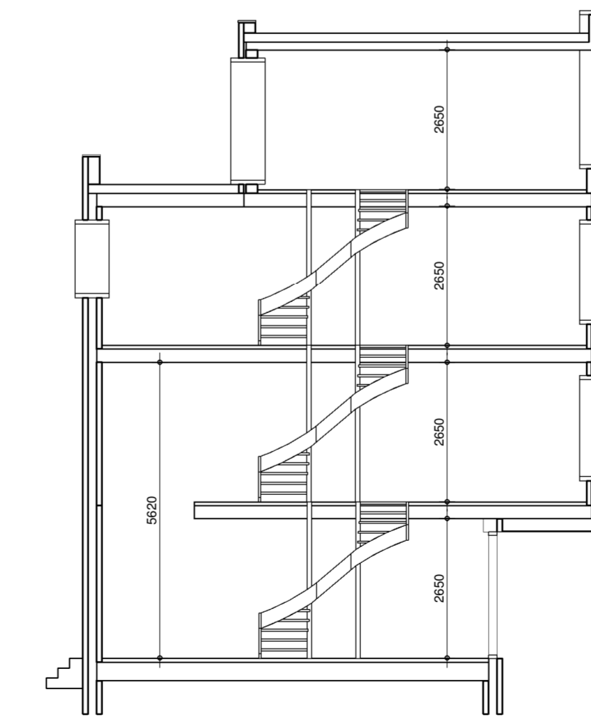
langsdoorsnede 1 : 100
