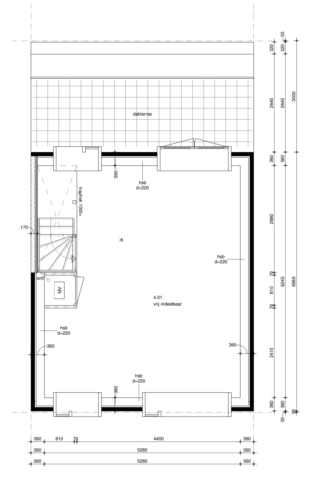
derde verdieping 1 : 50
