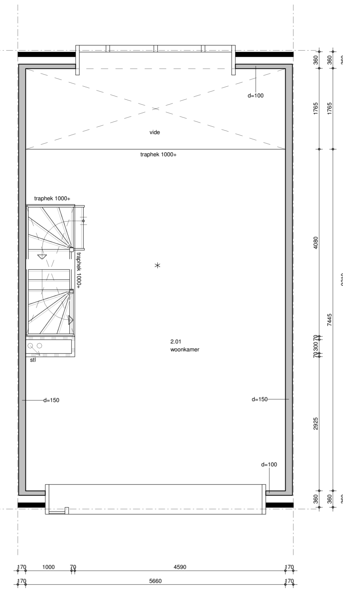
eerste verdieping 1 : 50
