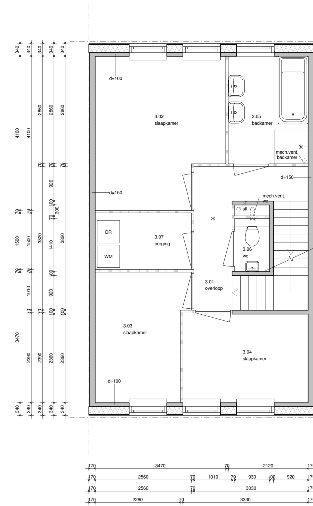
tweede verdieping 1 : 50
