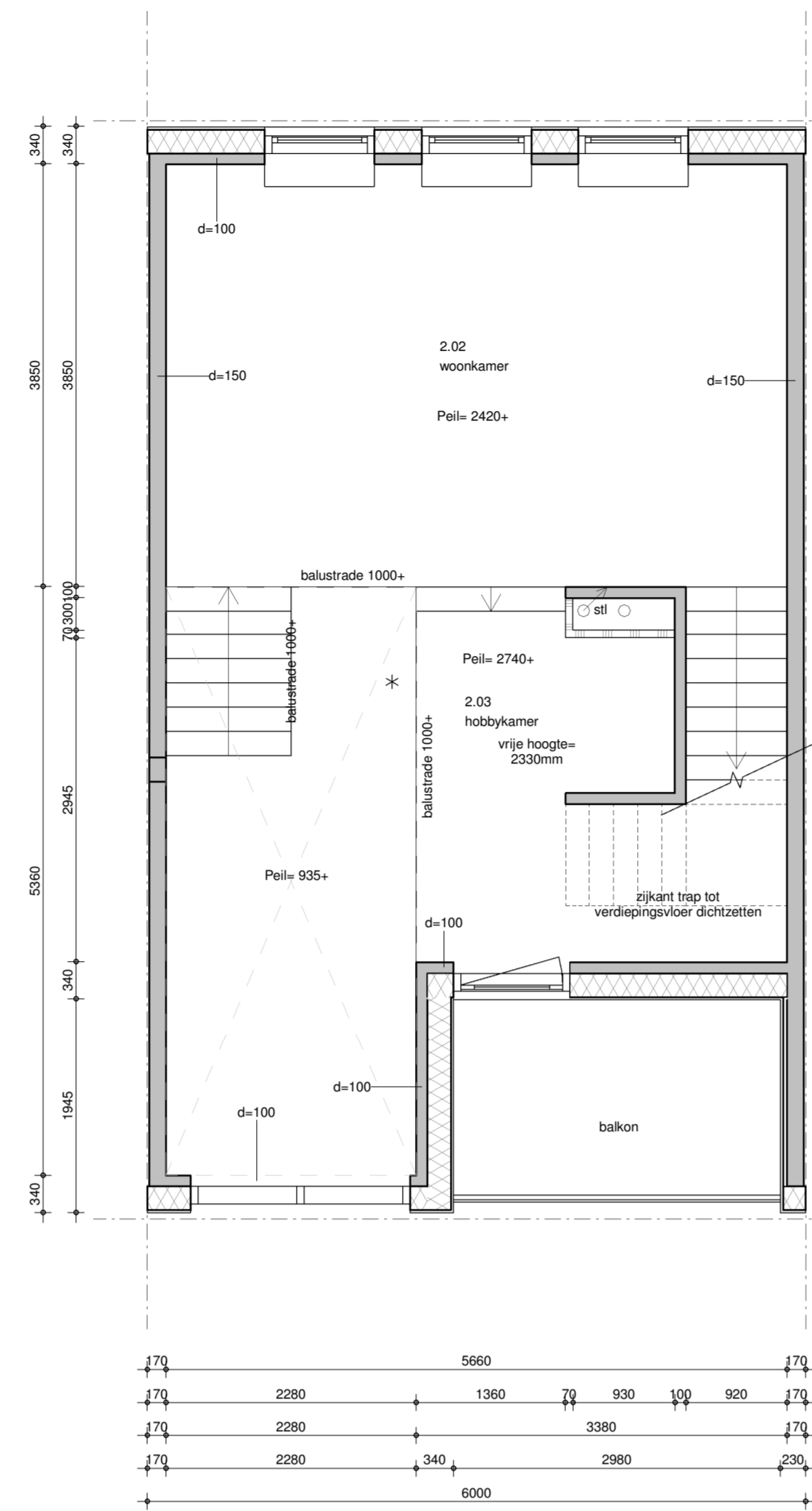
eerste verdieping 1 : 50
