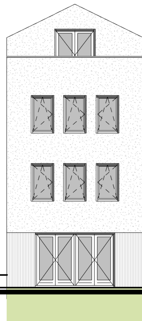
achtergevel 1 : 100
