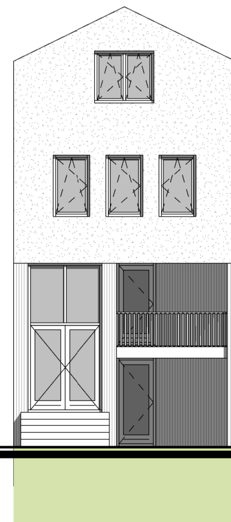
voorgevel 1 : 100
