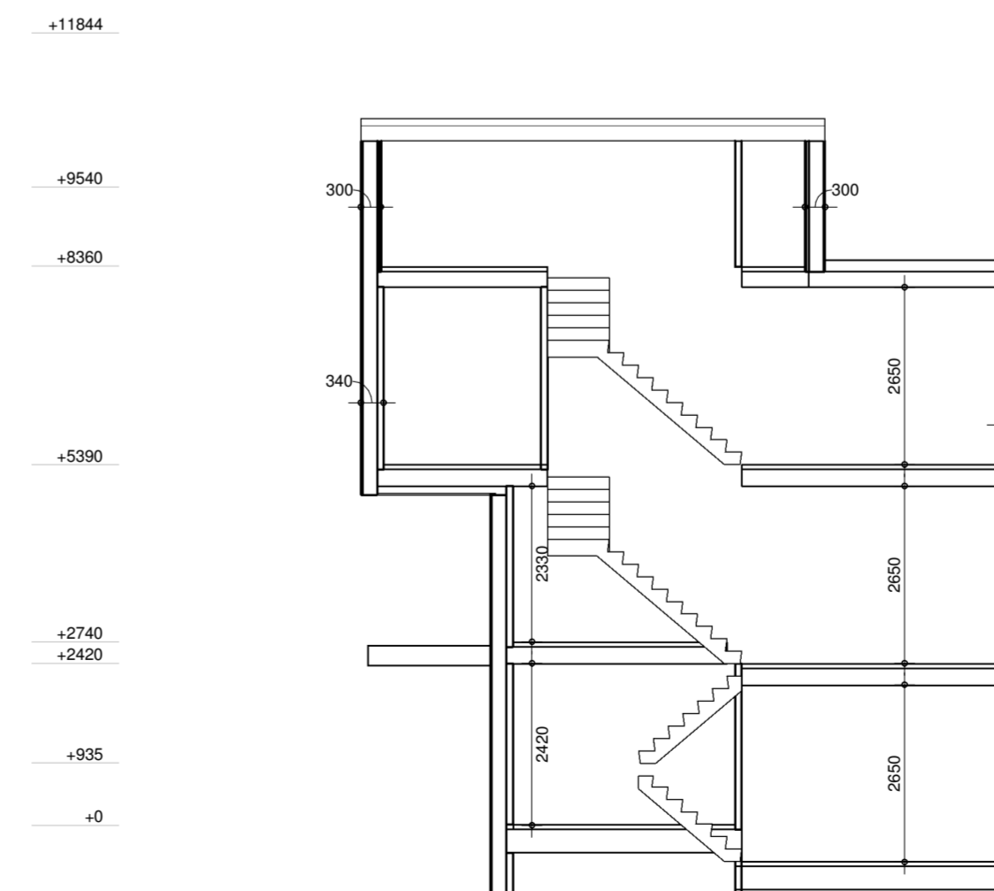
langsdoorsnede 1 : 100
