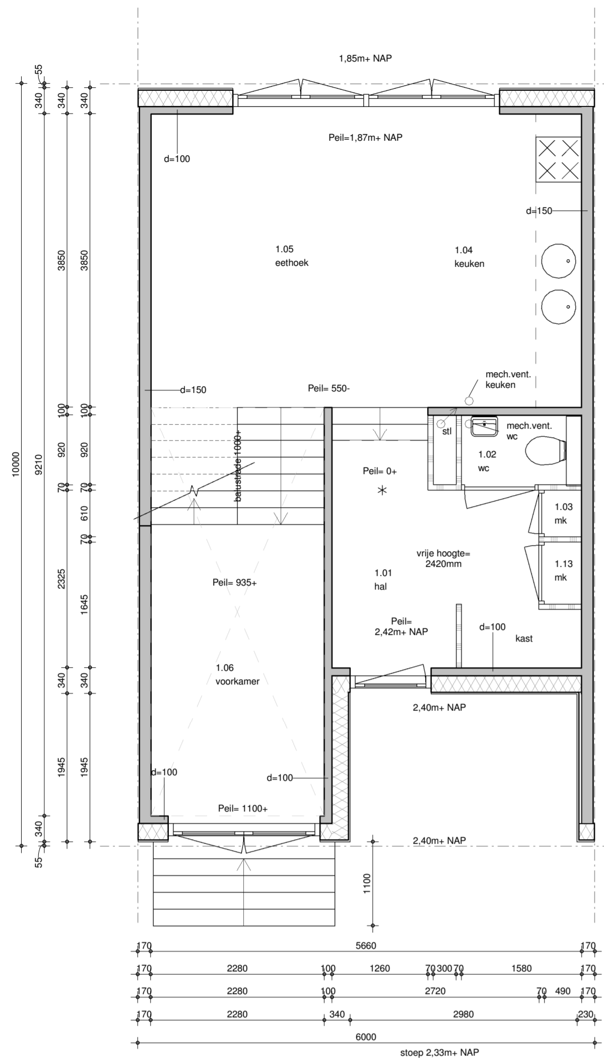
begane grond 1 : 50
