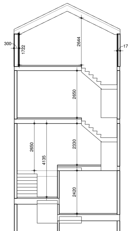
dwarsdoorsnede 1 : 100
